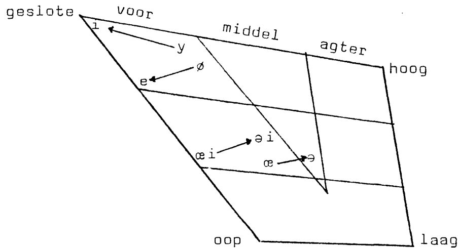
Figuur 2: vokaalkaart Geronde en ontronde allofoonpare in Kaapstadse Kleurling- Afrikaans
