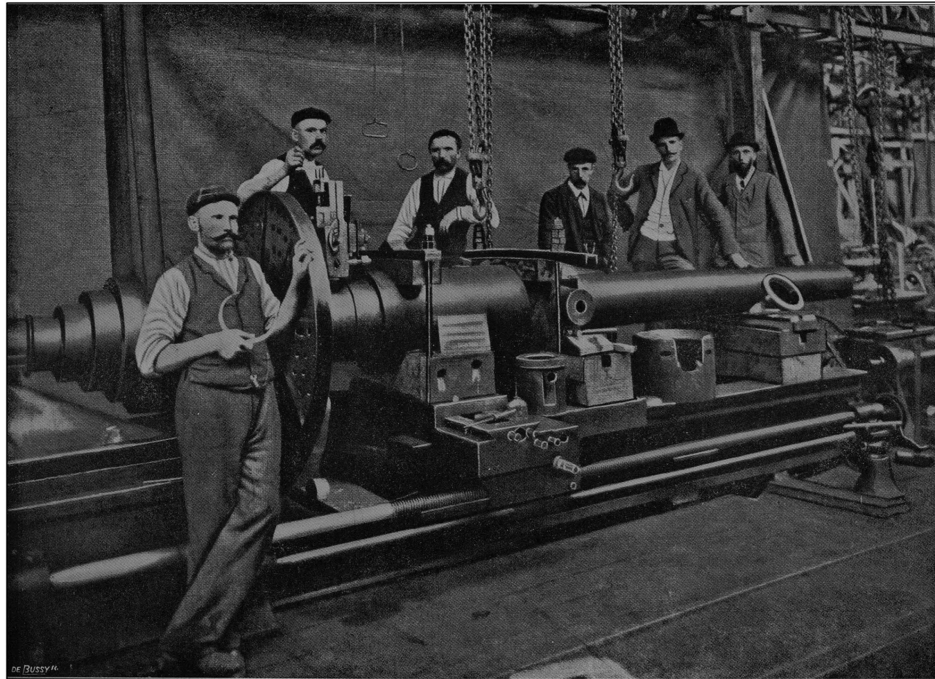
HET 15\frac{1}{2} C.M. CREUSOT-KANON, BIJGENAAMD „LONG TOM”, IN DE CENTRALE WERKPLAATS DER N. Z. A. S. M. TE PRETORIA. DE GEDELTEN, DIE VÓÓR EN ACHTER ZIJN AFGESNEDEN, LIGGEN ER VOOR.
