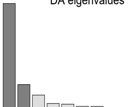
DA eigenvalues
