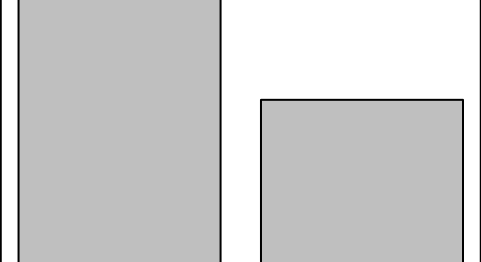
DA eigenvalues
