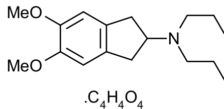
U 99194 maleate
