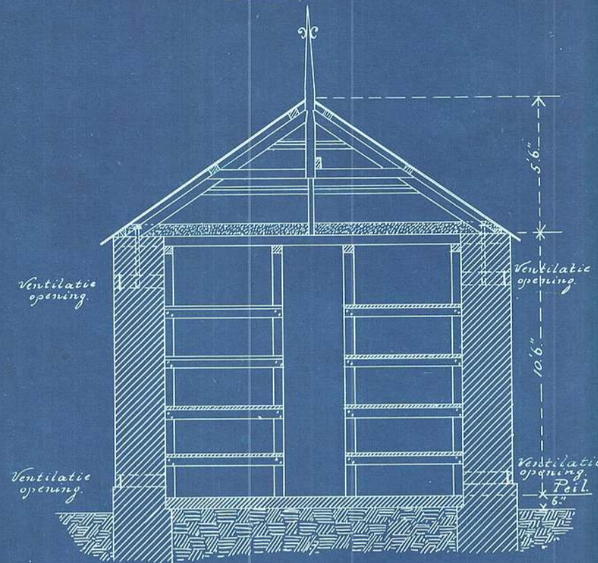
Doorsnede.
