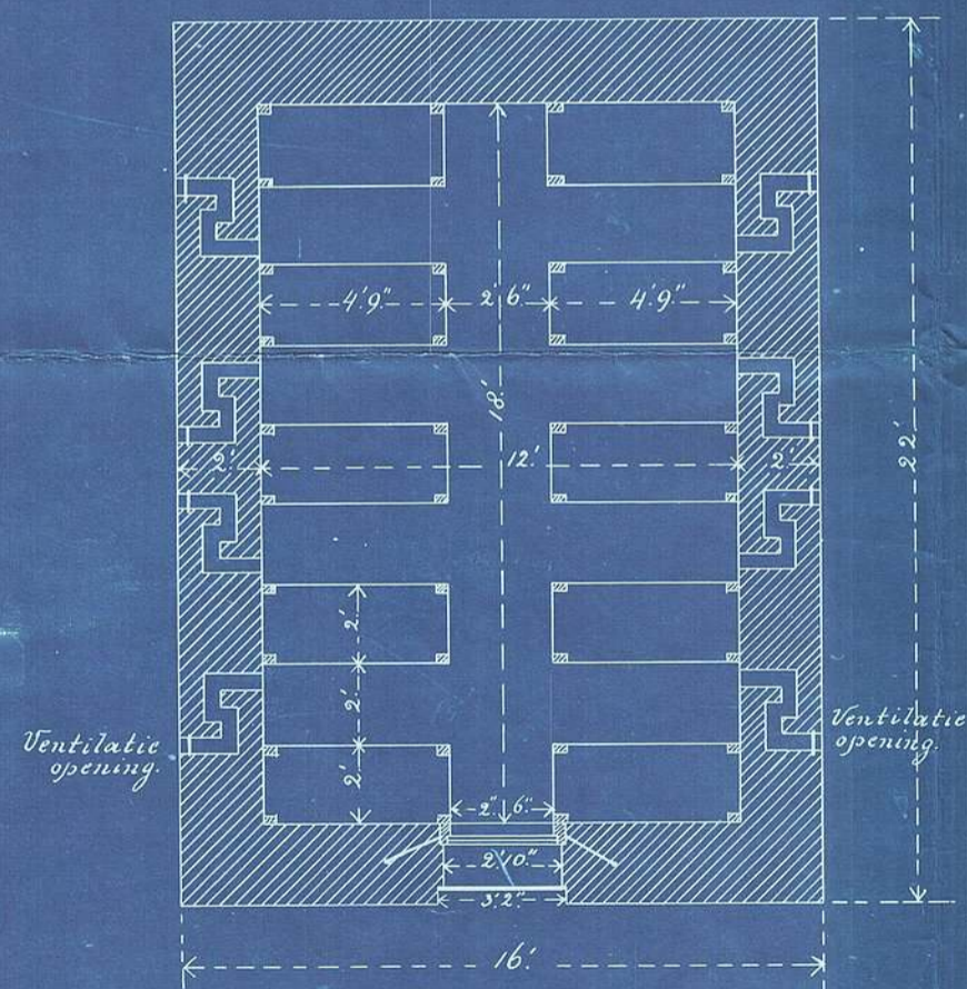
Platte grond.
