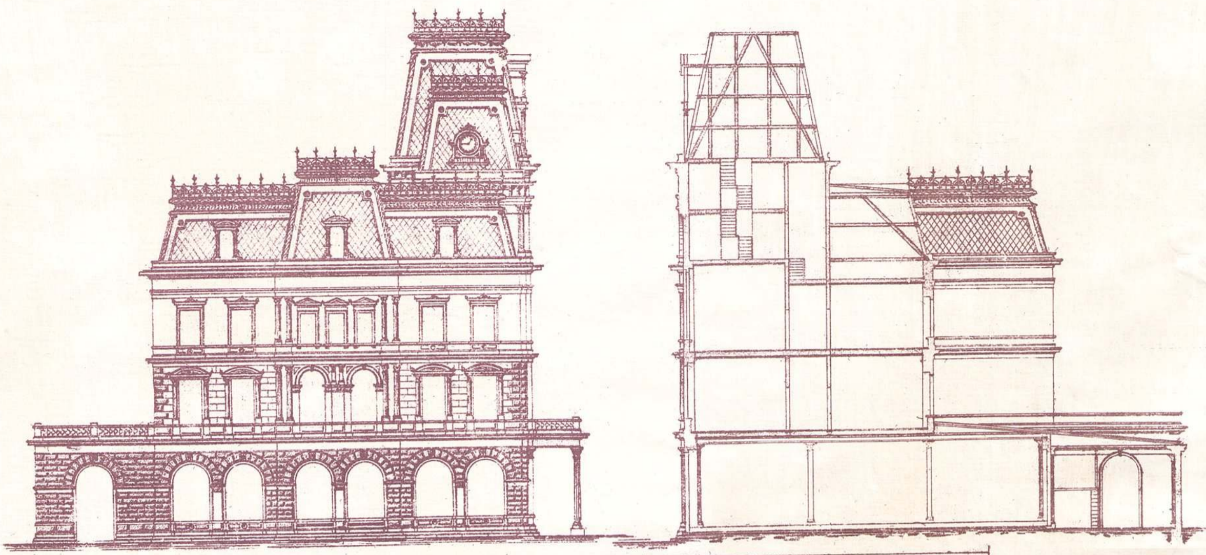
DOORSNEDE.
