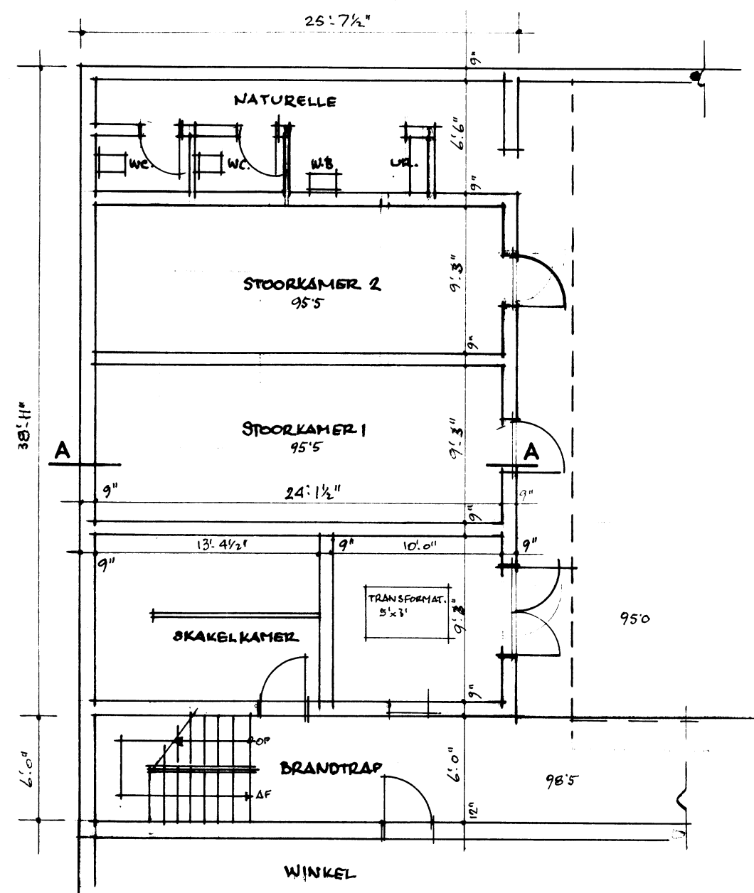
GRONDVLOERPLAN STOORKAMERS TWEDE VOORBEELD
