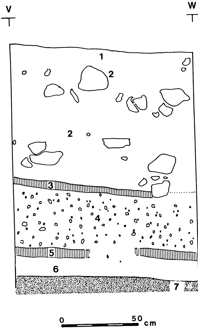
FIG 10 PROFIEL V - W
