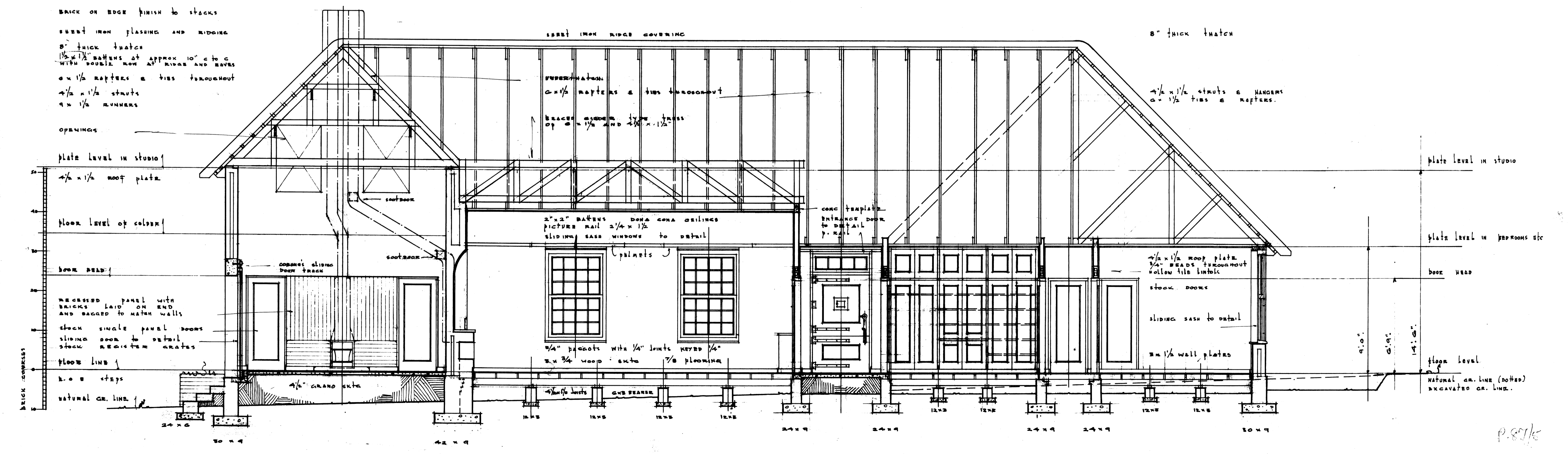
LONGITUDINAL SECTION AA
