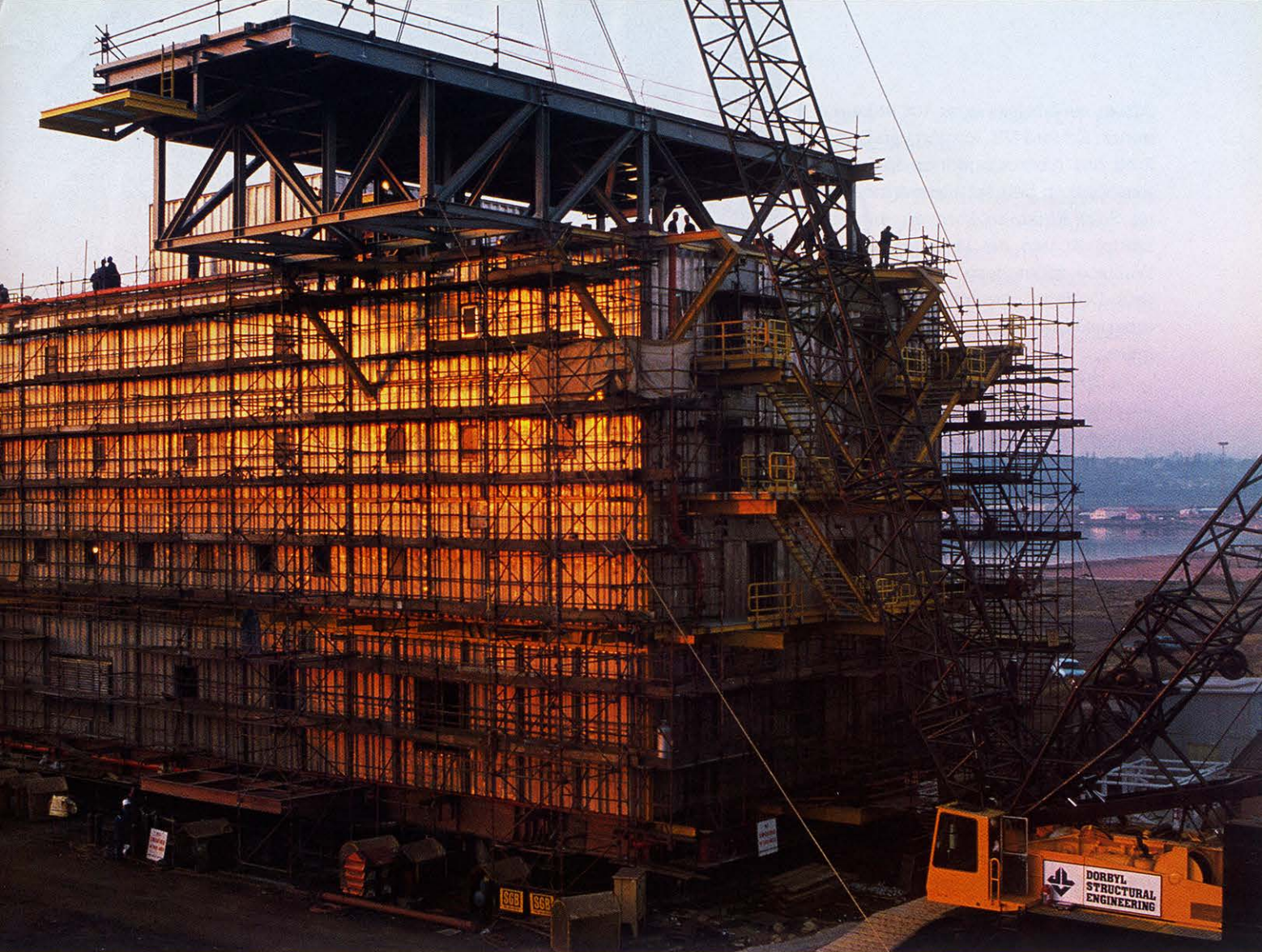
Die heliport word in posisie geplaas op die Mossgas-akkommodasie-module. Die hele eenheid is deur Dorbyl Shipbuilders in Durban gebou
