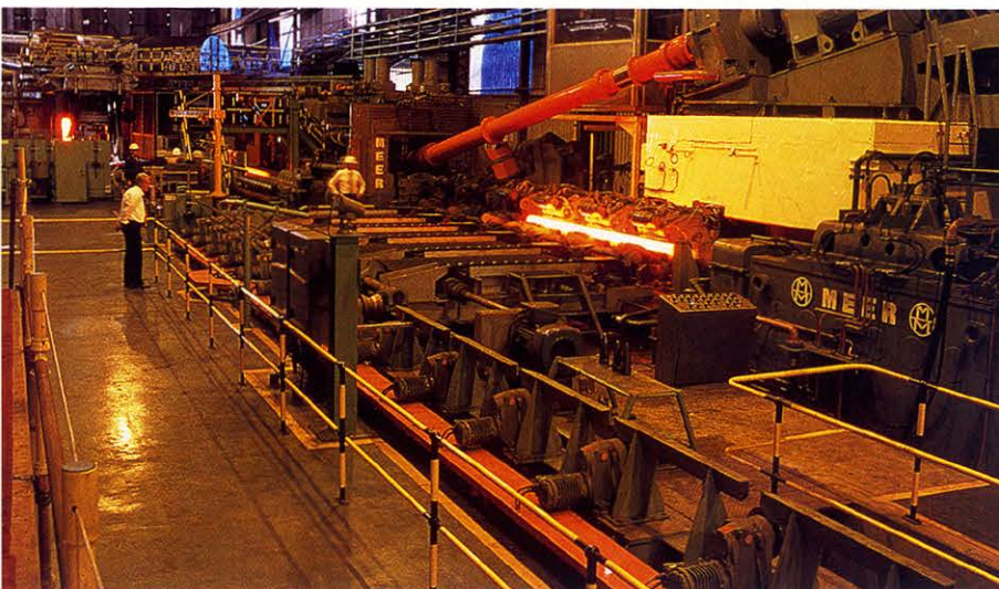
Tosa se nuwe walswerk in Vereeniging wat sy produksievermoë van naatlose pype van 22 000 tot 60 000 ton per jaar sal opstoot
