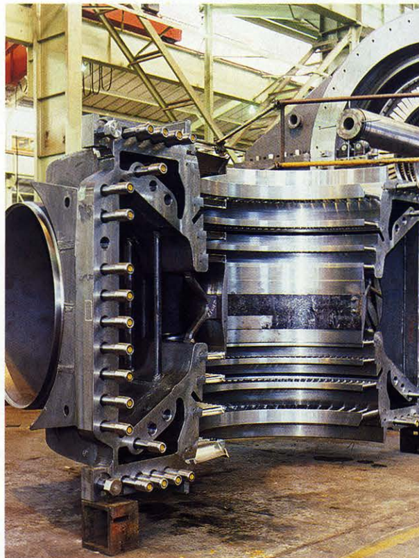
'n Gegote en gemasjineerde turbinekomponent vir die Kendalkragentrale in Oos-Transvaal, wat deur Dorbyl se Broderick-werke vervaardig is
