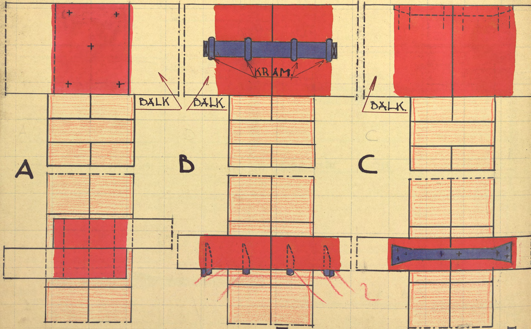
FIG 13 OP 1/3 WG.
