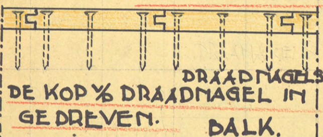
FIG 17 OP 1/5 W.G.
