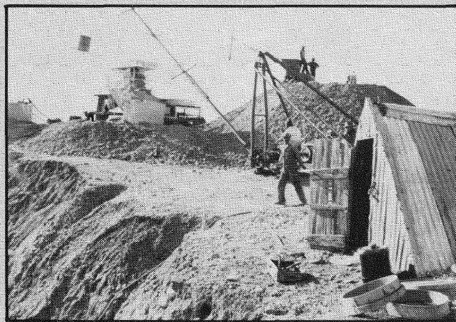
Op die kleim. Hyskraan vir diep delf. Sinkkaia regs voor.
