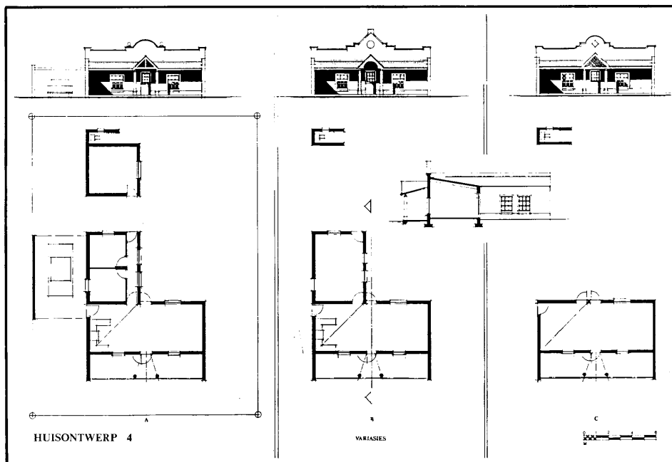
TEKENING 6: Aansigte en planne van 'n invulhuis waar verskeie alternatiewe aangetoon word. (P. Cooper)
