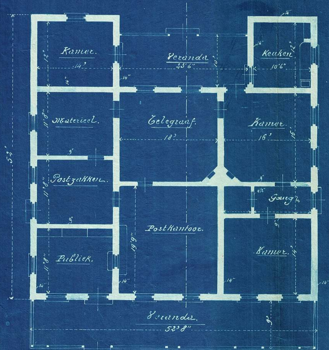
Grondplan.
