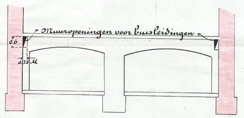
Doorsnede CD.
