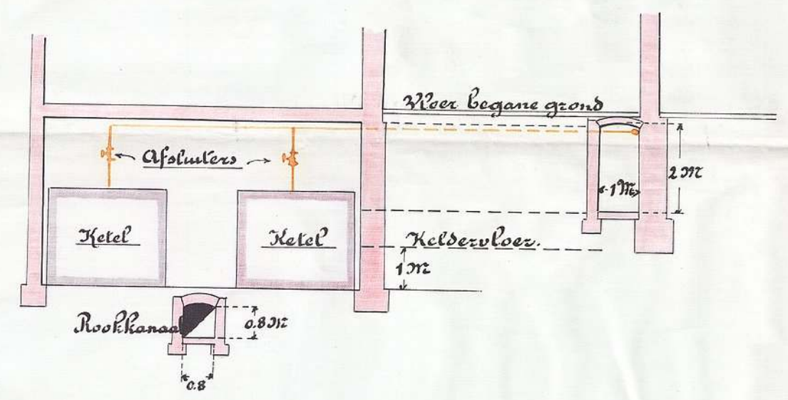
Doorsnede AB (Ketelruis en buisleidingen)
