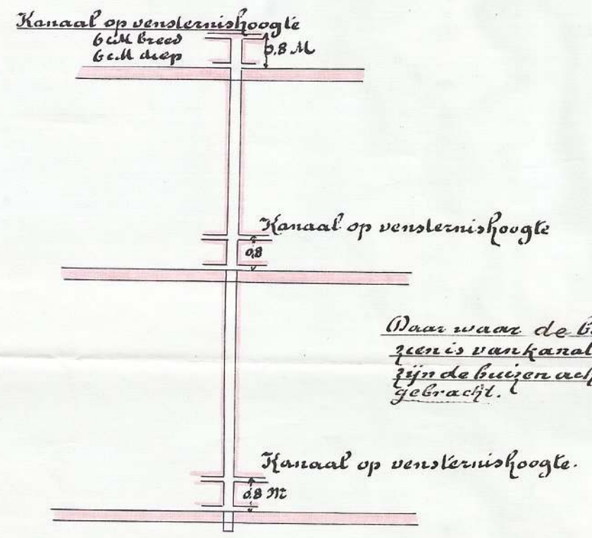
Muursleuf voor verticale buizen.
