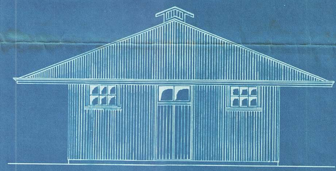
Zijgevel.
