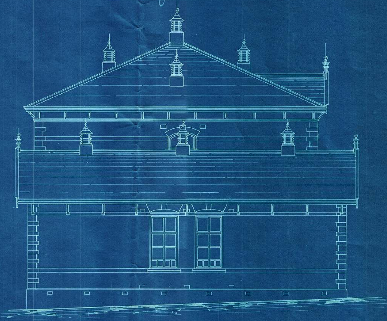
Eindgevel
