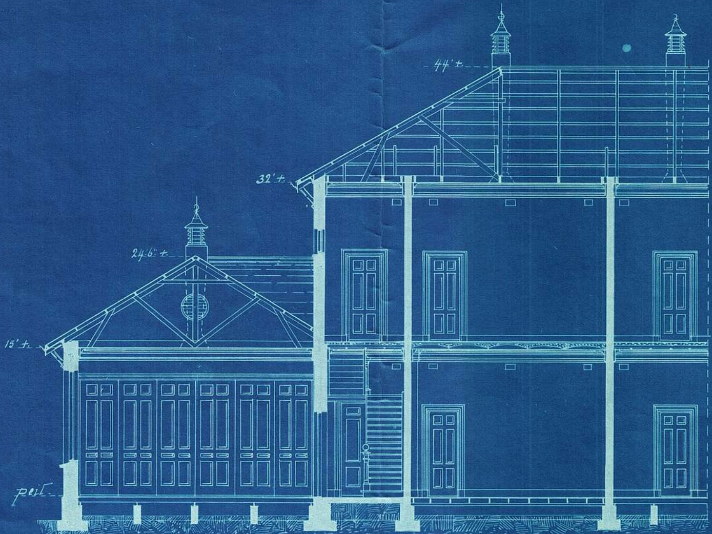
Doorsnede A. B.
