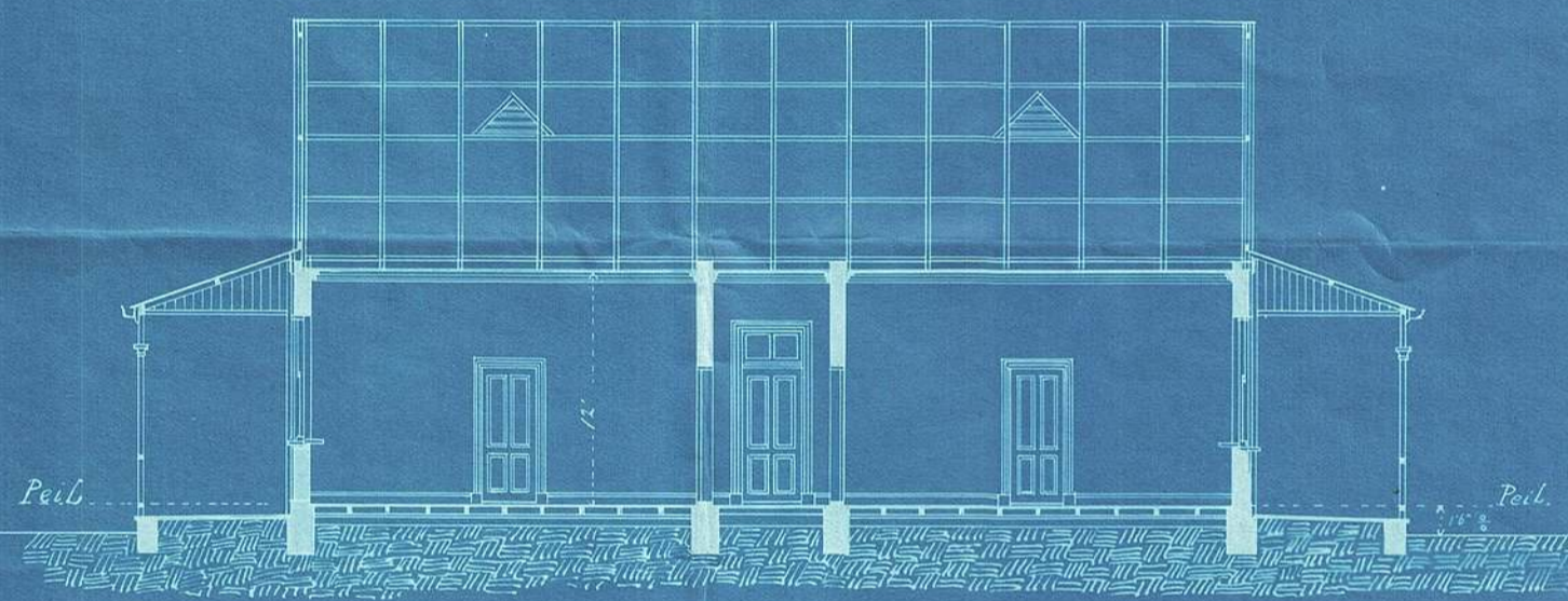
Doorsnede C. D.
