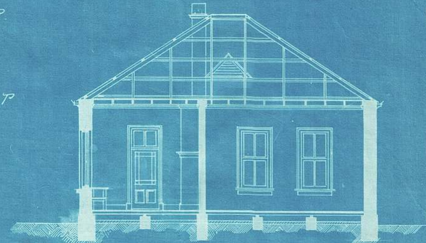
Doorsnede C-D.
