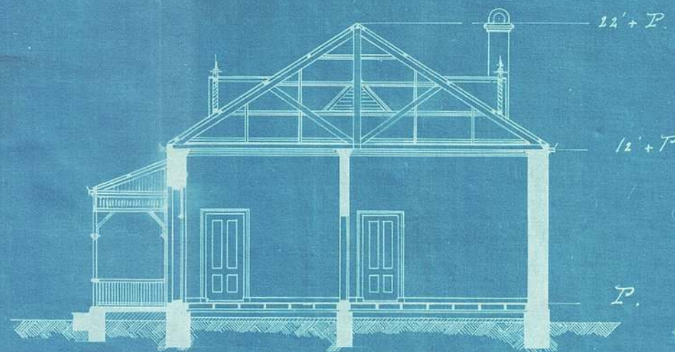
Doorsnede A-B.
