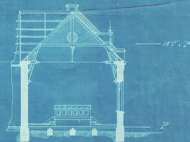
Doorsnede G-H.
