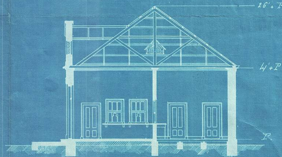
Doorsnede E-F.
