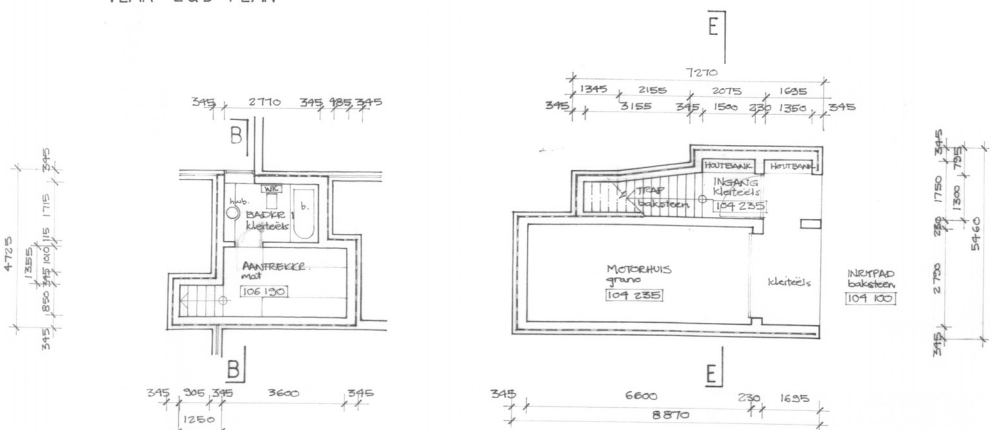
BADKR 1 PLAN
