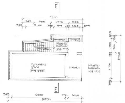
VLAK 1 PLAN
