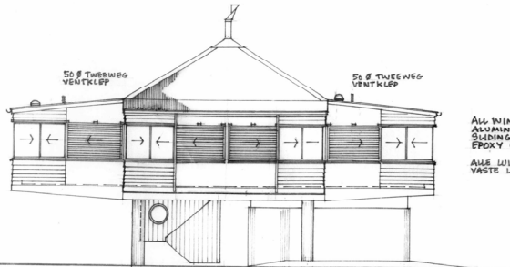
SUID-AANSIG 1:100
