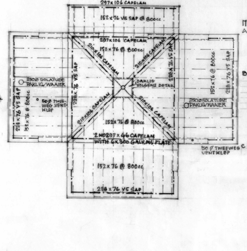
DAK-PLAN 1:100
