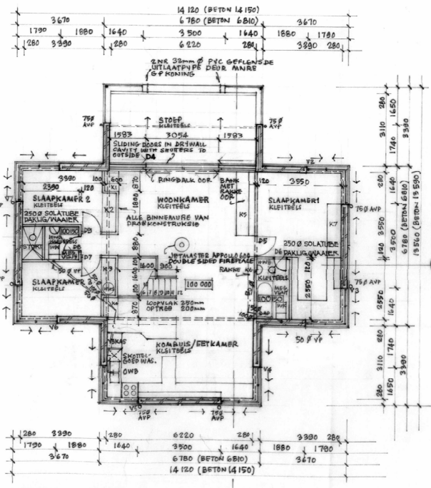
EERSTEVLOER-PLAN 1:100
