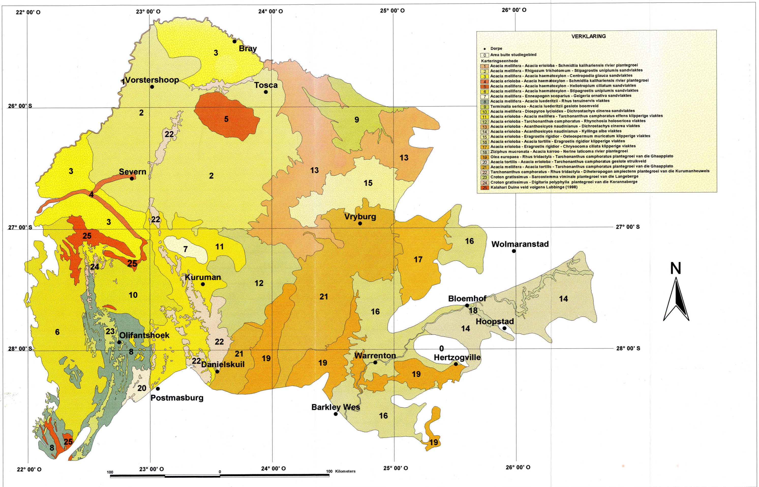
Figuur 17. Plantegroeikaart van die suidoostelike Kalahari Doringveld
