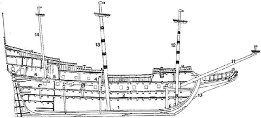
Figuur 6: Snit deur 'n tipiese spiegelretourschip
