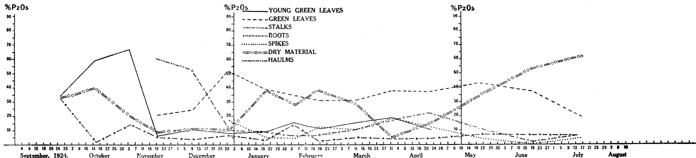
CHART 17.— Cymbopogon plurinodis .
