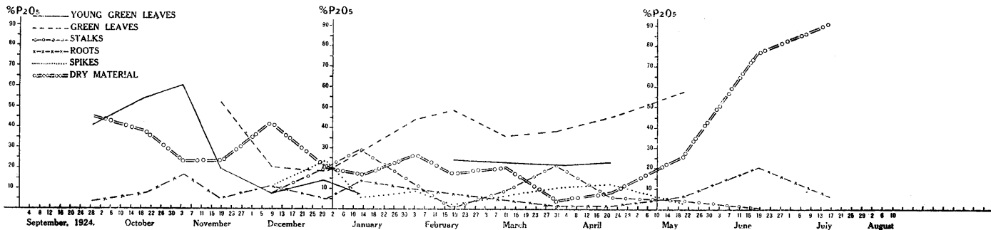
CHART 24.— Anthephora pubescens .
