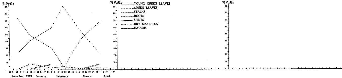
CHART 26.— Tragus racemosus .
