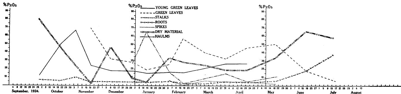
CHART 15.— Digitalia eriantha .
