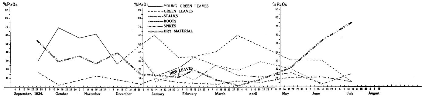
CHART 18.— Pogonarthria falcata .
