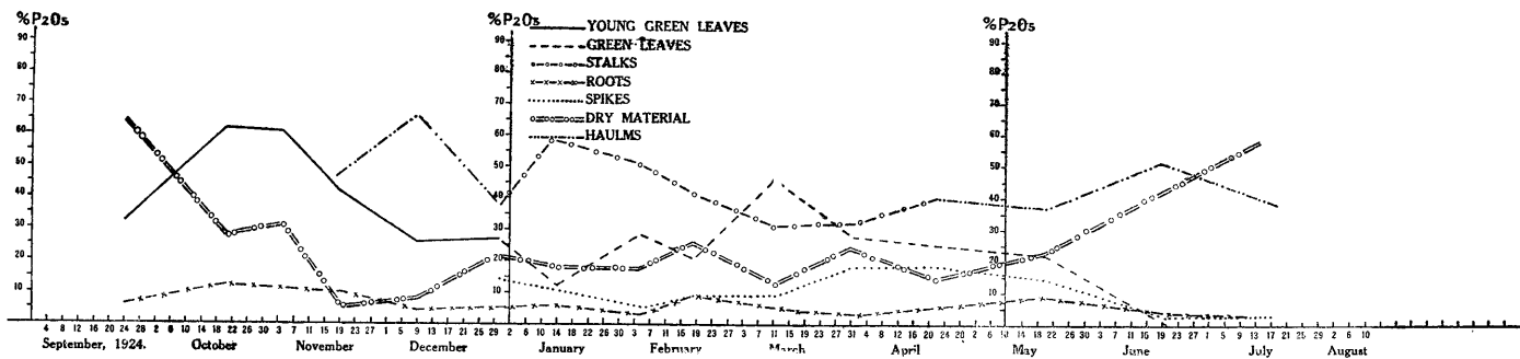
CHART 23.— Aristida uniplumis .
