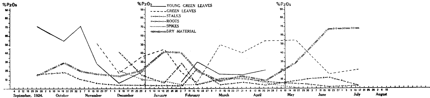
CHART 21.— Sporobulus fimbriatus .
