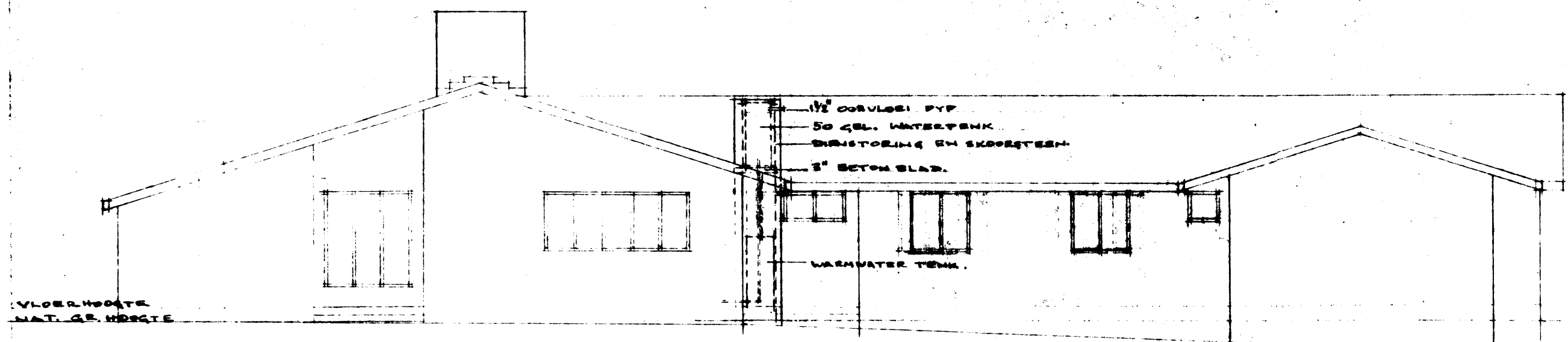
SUID AANSIG.
