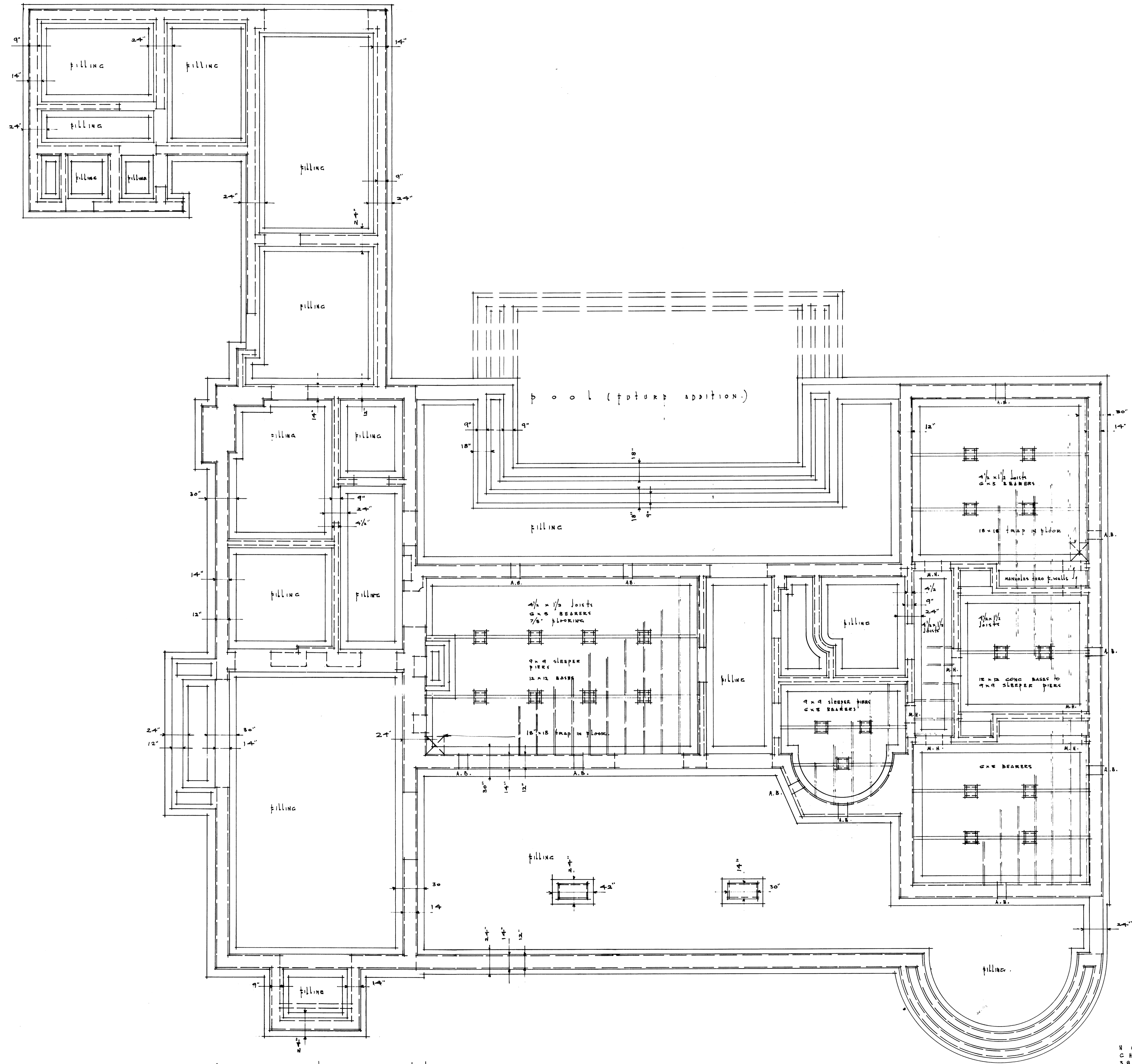
F O U N D A T I O N P L A N
