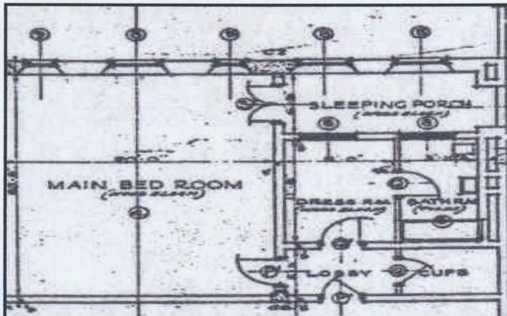
Figuur 95: Die oorspronklike planne vir die hoofslaapkamer van Libertas
