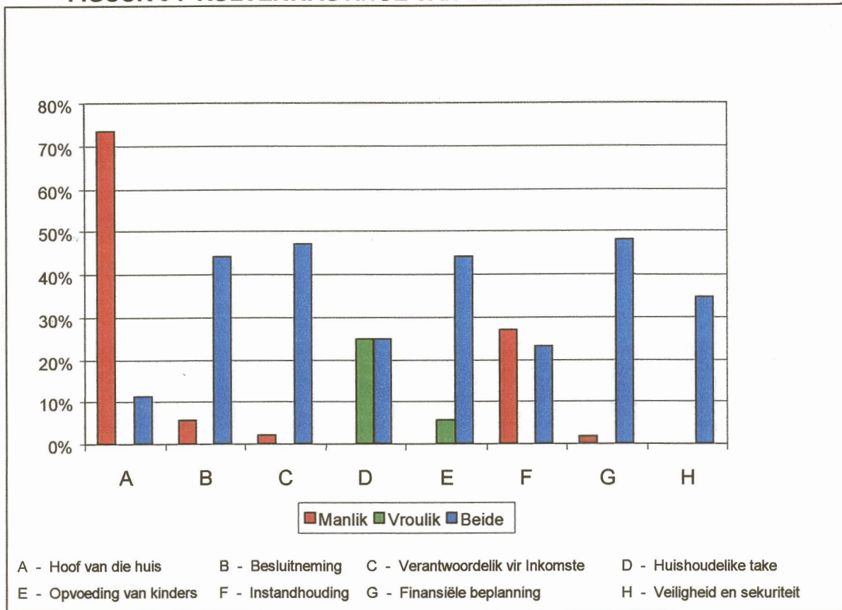
FIGUUR 3 : ROLVERWAGTINGE VAN DIE MANLIKE RESPONDENTE
