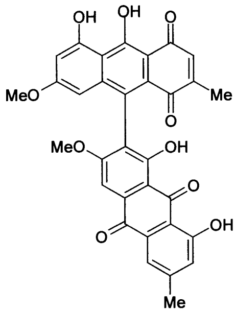
Isosengulone
