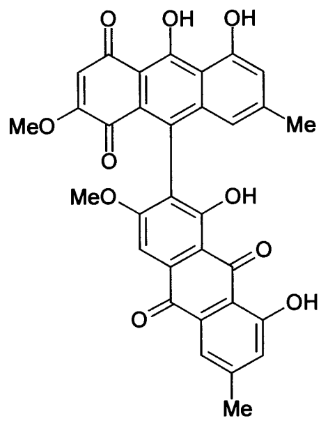
Sengulone
