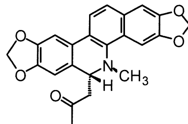
8-acetyldihydroavicine
